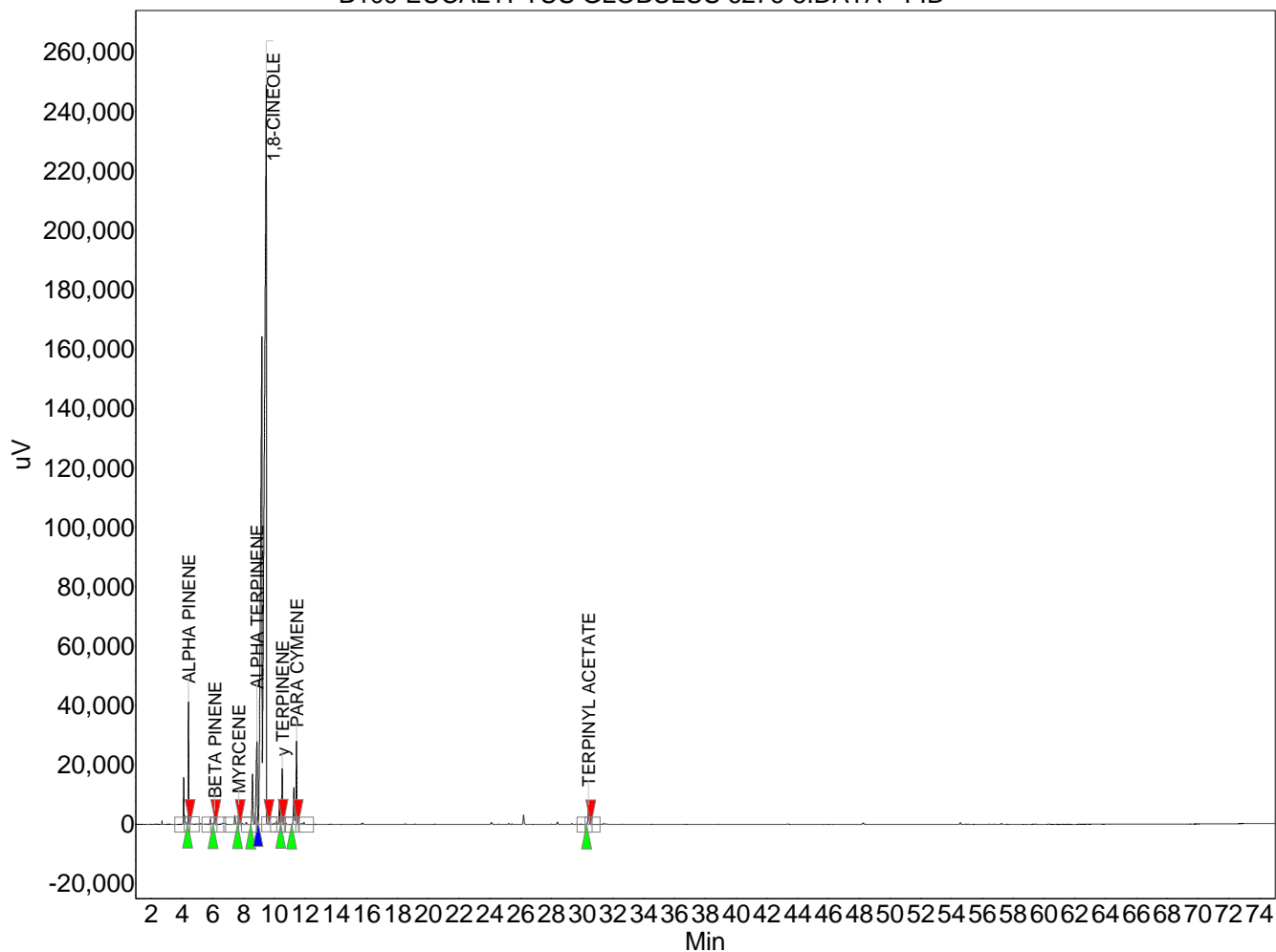
B109 EUCALYPTUS GLOBULUS 6276-5.DATA - FID
